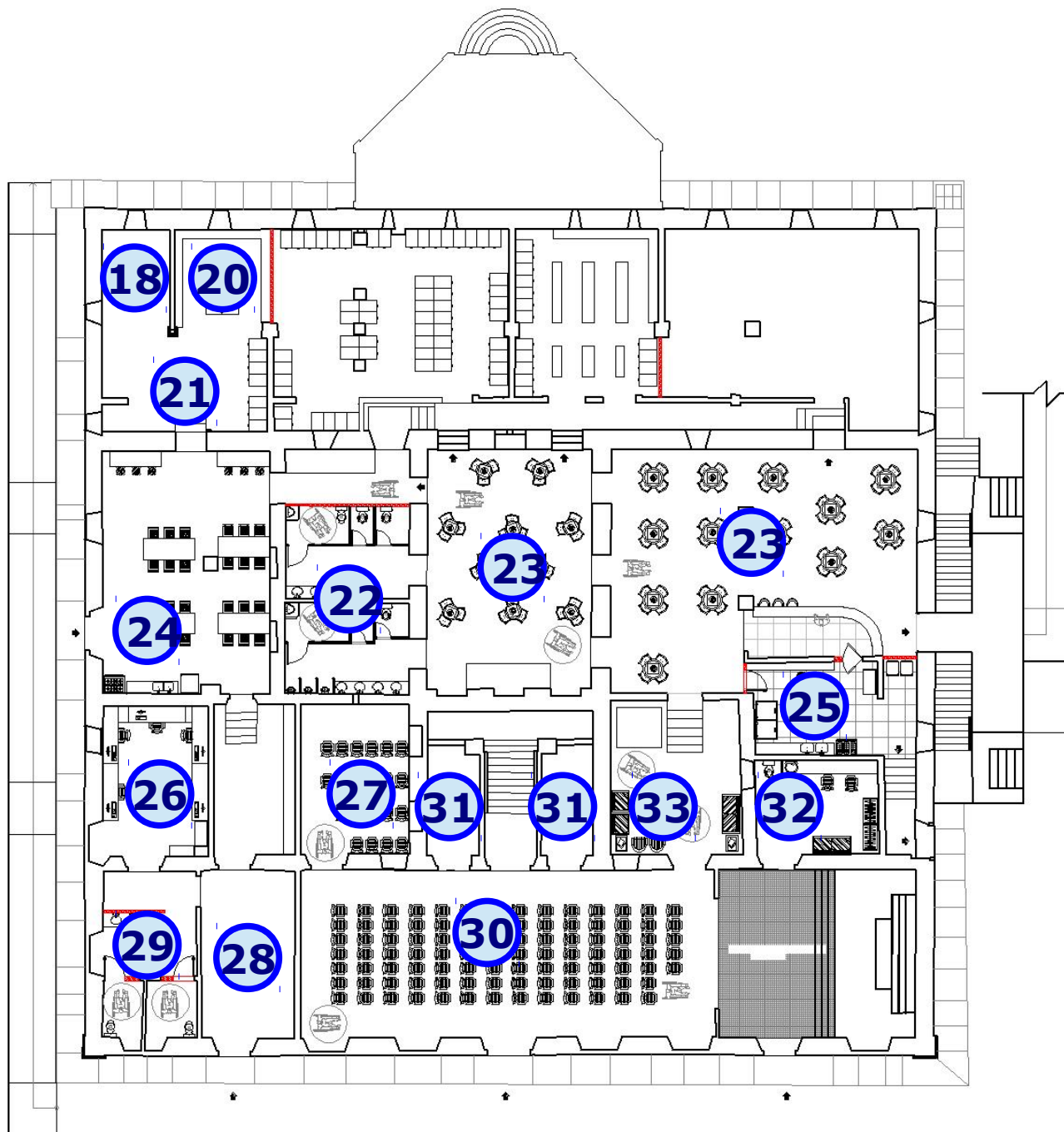
Planta Baixa Pavimento Inferior
